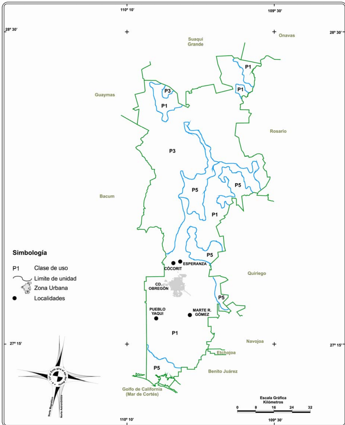
Mapa 17. Uso potencial Pecuario del Municipio de Cajeme
