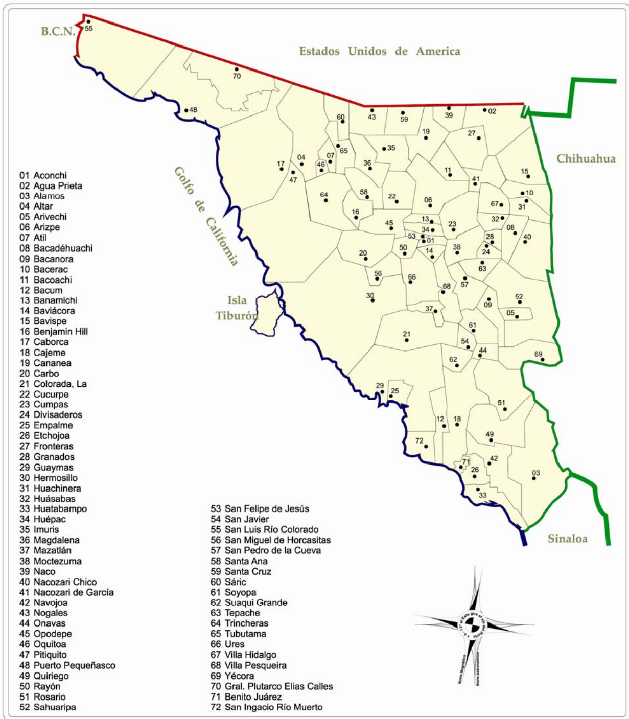
Mapa 2. División Política del Estado de Sonora
