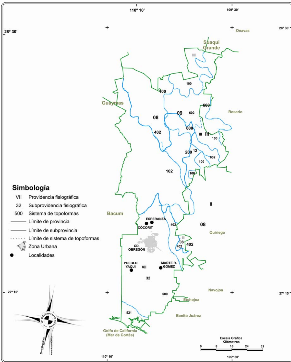
Mapa 9. Fisiografía del Municipio de Cajeme
